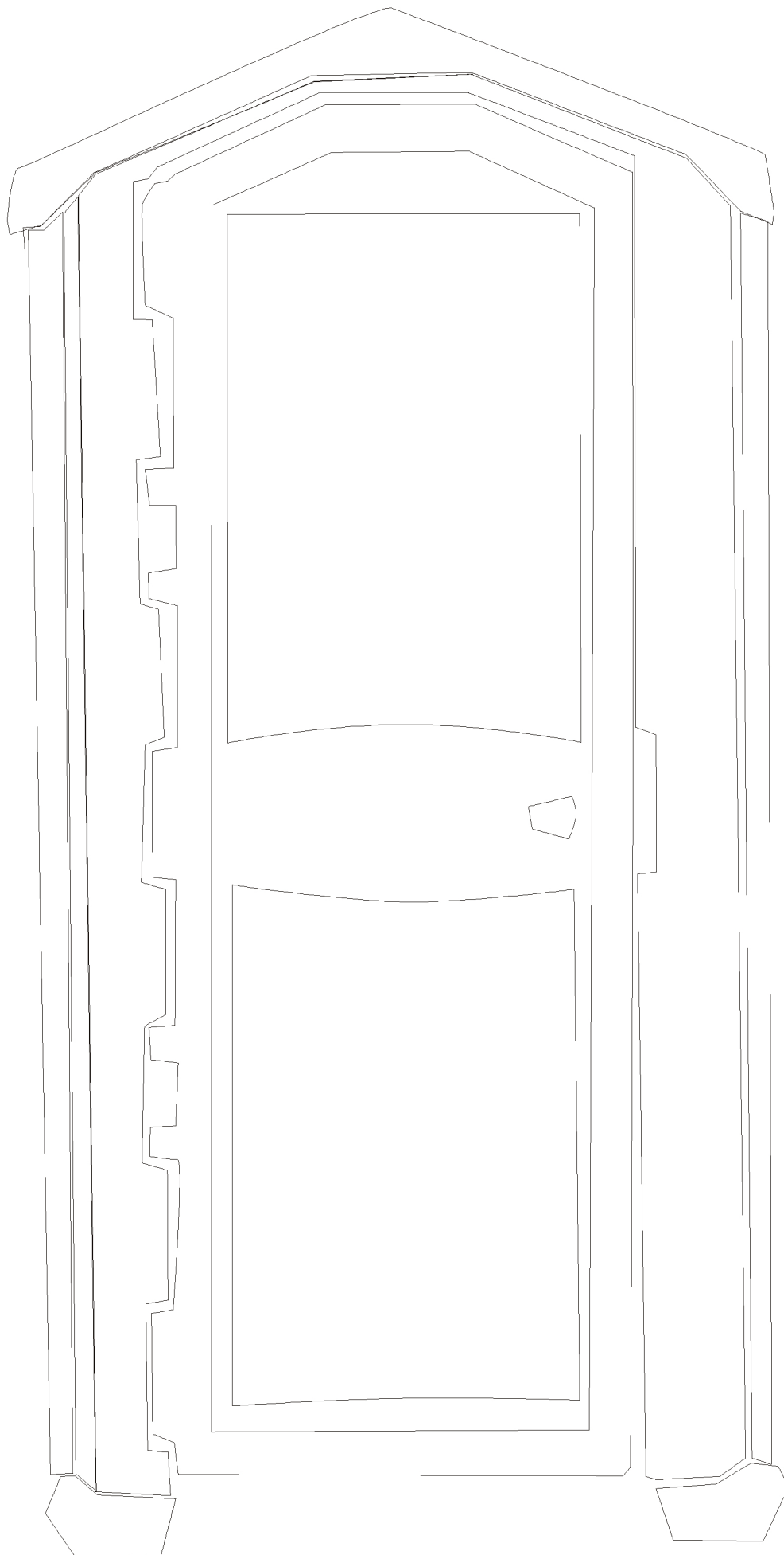
Front-Ansicht einer WC-Kabine Maße: Höhe 2,10m, Breite:1,12m
